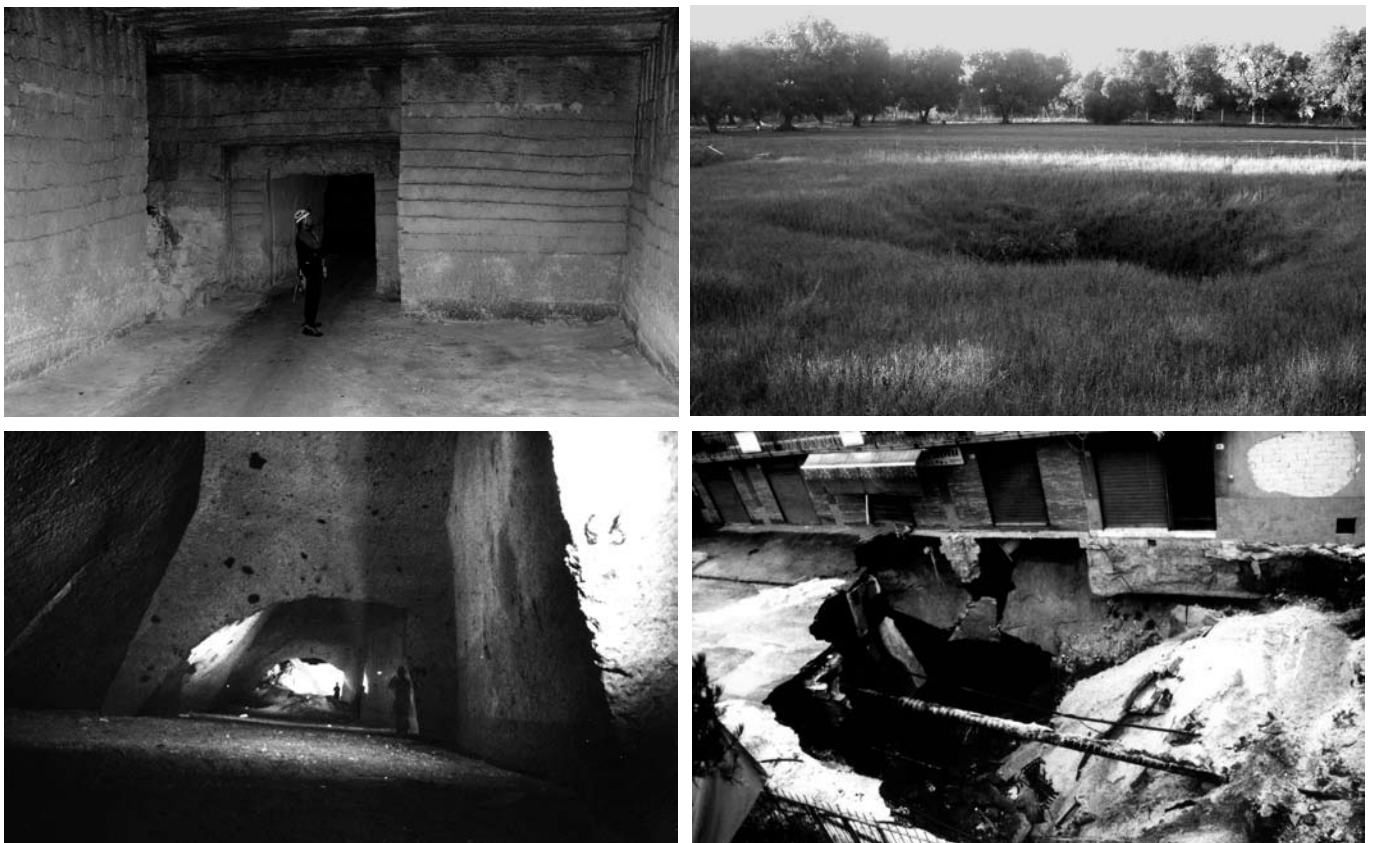
Fig. 19 - Esempi di cavità sotterranee che hanno dato luogo a fenomeni di sprofondamento (Cutrofiano, in alto, e Lusciano, in basso) talora provocando anche gravissimi danni al tessuto rurale e urbano sovrastante (foto di Cutrofiano: M. Parise; foto di Lusciano: B. Bocchino, S. Del Prete).
