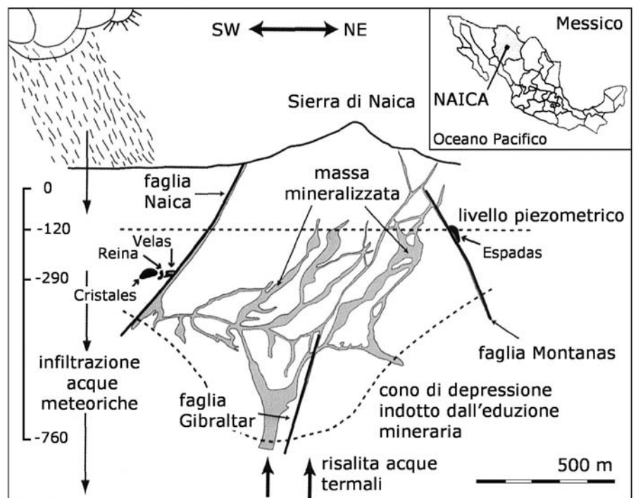
Fig. 7 - Miniere di Naica: l'abbassamento indotto della falda permette lo sfruttamento della massa mineralizzata con la conseguente realizzazione di gallerie minerarie a profondit  sempre maggiori (da Forti, 2006, modificato da Lang, 1995). Nel momento in cui termineranno i lavori estrattivi e la falda ritorner  al suo livello piezometrico normale, le gallerie realizzate verranno gradualmente sommerse.
