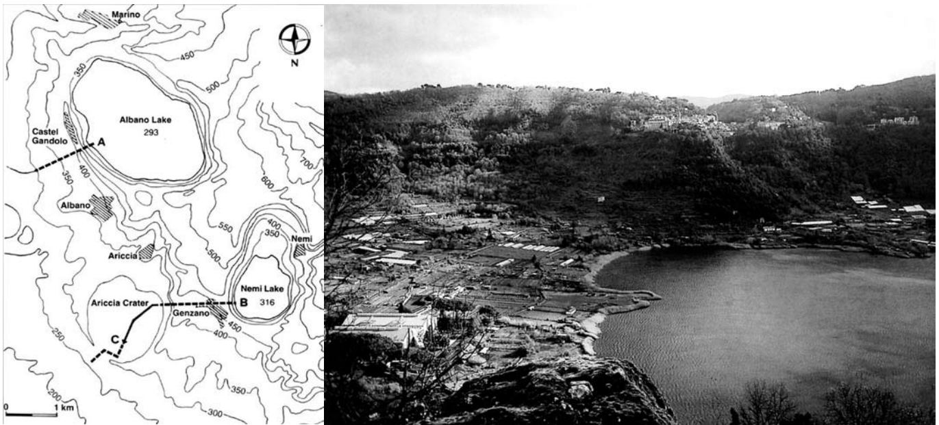
Fig. 8 - Schema topografico delle conche endoreiche di origine vulcanica dei Colli Albani nel Lazio con il tracciato dei relativi emissari (da Castellani e Dragoni, 1989). A destra una panoramica del Lago di Nemi (foto: C. Germani).
