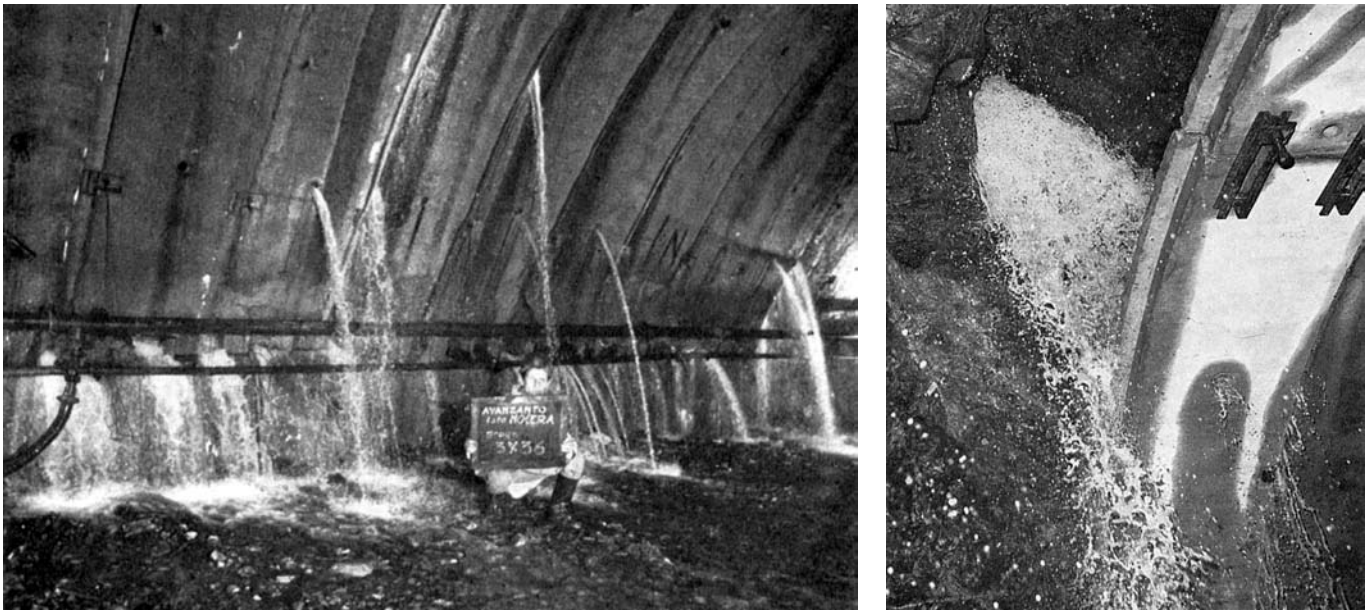
Fig. 6 - Venute d'acqua durante le fasi di avanzamento della galleria ferroviaria S. Lucia nel tratto Nocera - Salerno (da Celico et al., 1977).
